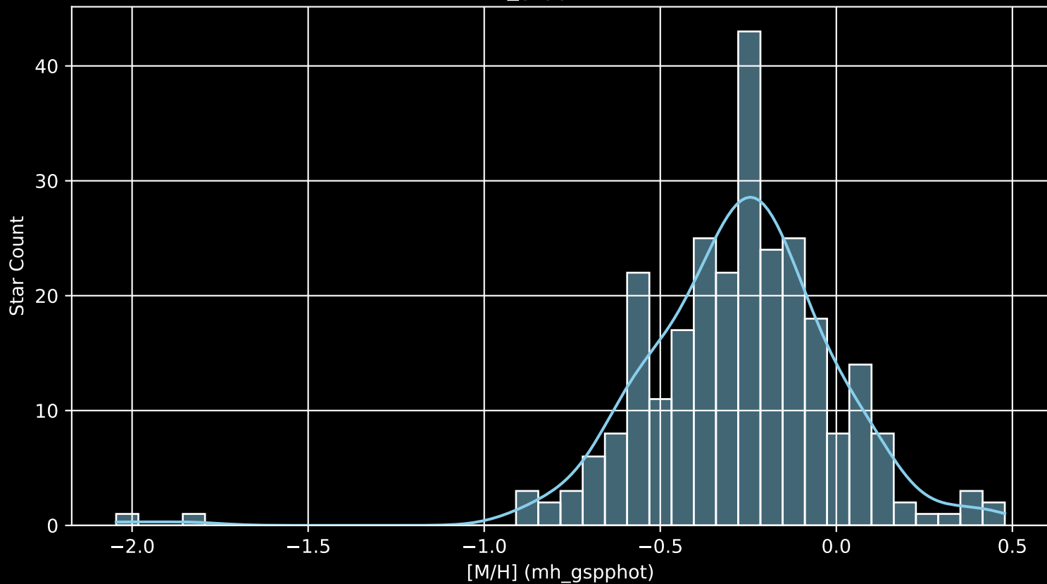
GALAH DR4 Field: [2485] [M/H] (mh_gspphot) (n= 270)
