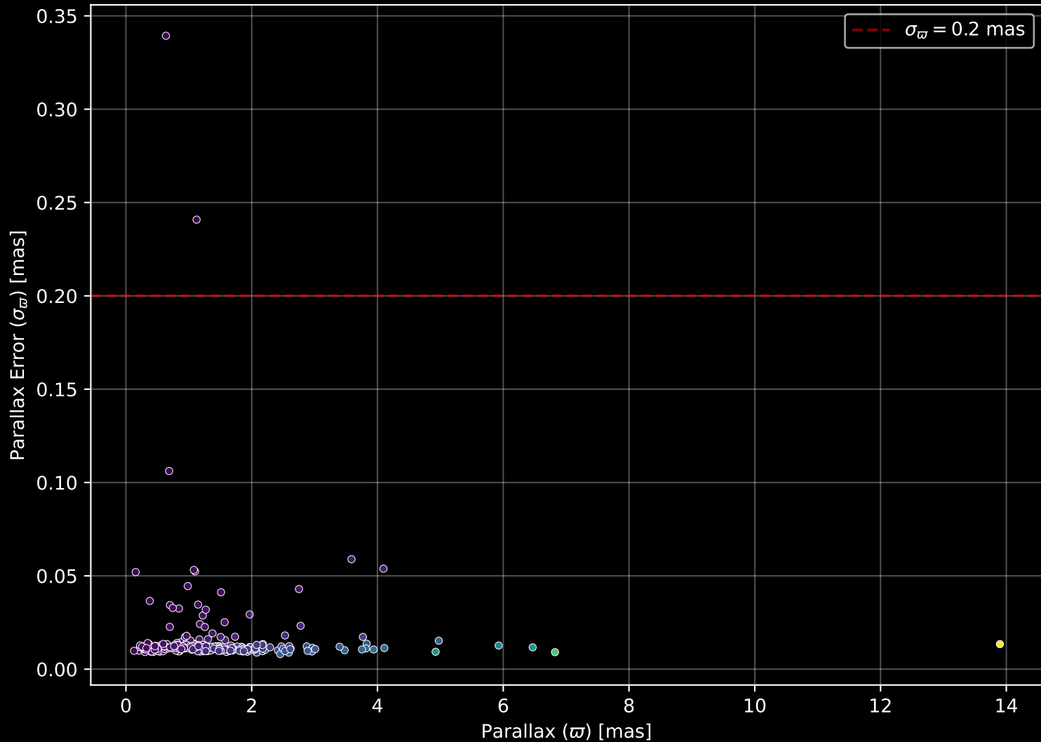
GALAH DR4 Field: [2485] Parallax Quality (n= 270)
