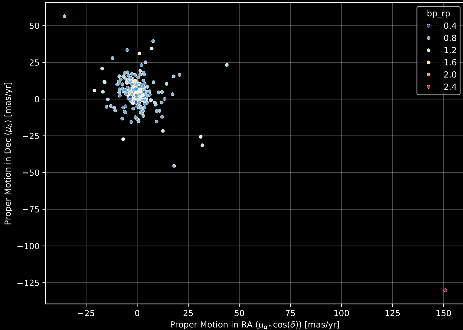
GALAH DR4 Field: [2485] Proper Motion Diagram (n= 270)
