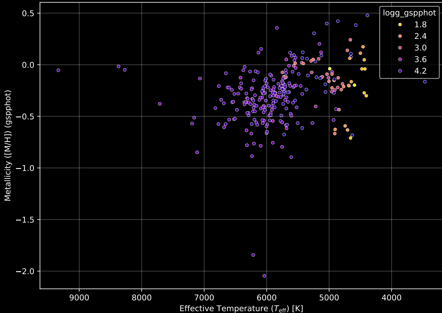
GALAH DR4 Field: [2485] Stellar Population Parameters (n= 270)
